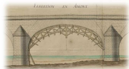
Quelques archives des plans de la construction du pont...
